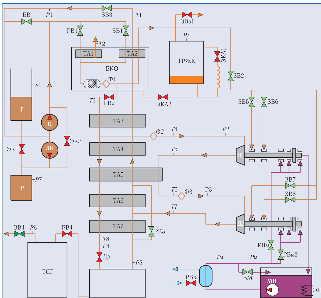
Рис. 2. Принципиальная схема турбодетандерного ожижителя гелия с элементами САУ: Г — газгольдер; К — технологический компрессор; ЗК — закачной компрессор; Р — ресивер; Д1, Д2 — детандеры; МН — масляный насос; БКО — блок криогенной очистки гелия; ТСГ — гелиевый сосуд Дьюара; ТРЖК — азотный сосуд Дьюара; ТА1-ТА7 — теплообменные аппараты; Ф1-Ф3 — фильтры; ЭП — электроподогреватель; ЭКГ — электроклапан пополнения газгольдера; ЭКЗ — электроклапан закачки; ЭКА1 — электроклапан поддержания давления в азотном сосуде Дьюара; ЭКА2 — электроклапан подлива жидкого азота в азотную ванну КГУ; БВ — байпасный вентиль; БМ — байпасный вентиль маслонасоса; Др — дроссельный вентиль; ЗВ1-ЗВ8 — запорные вентили; РВ1-РВ4 — регулирующие вентили; P — давление; T — температура; У — уровень; цветом обозначено: коричневый — гелий, оранжевый — азот, сиреневый — масло; голубой — вода; красный — «закрыто», «заторможено», зелёный — «открыто», «работает»
